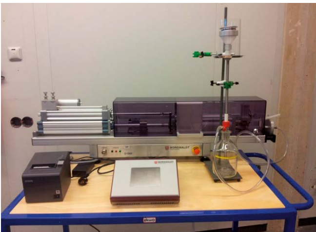
Laboratorium waterpijppopstelling
