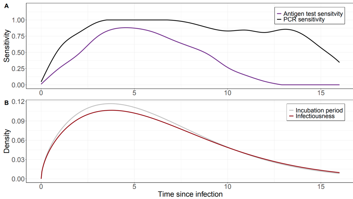
Figuur 2 Tijdsafhankelijke gevoeligheid, besmettelijkheid en incubatietijd 4 . (A) Tijdsafhankelijke testgevoeligheid voor antigeentest en PCR-test gebruikt in het model. (B) Incubatietijdverdeling en tijdsafhankelijke besmettelijkheidscurve gebruikt in het model.
