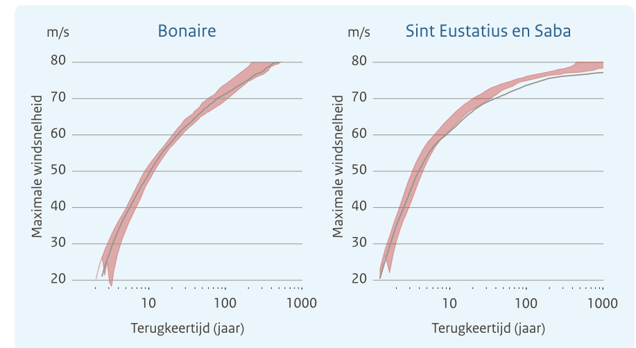
Figuur 30. Herhalingstijden van windsnelheden binnen 250 km van de BES-eilanden, nu (1980-2017, grijs) en in de toekomst (2015-2050, rood) bij het hoge uitstootscenario.
