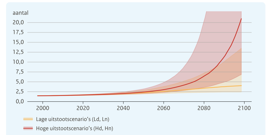
Figuur 44. Aantal sluitingen van de Oosterscheldekering, gebaseerd op berekeningen van het zeeniveau in twee KNMI'23-klimaatscenario's en de aanname dat het sluitpeil van de kering, drie meter boven NAP, gelijk blijft.
