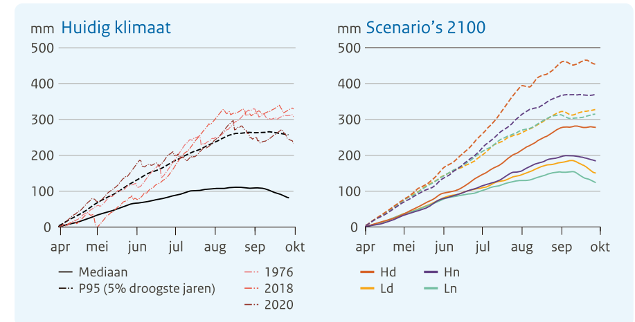
Figuur 17. Doorlopend cumulatief neerslagtekort in De Bilt in het huidige klimaat (1991-2020) (links) en rond 2100 voor de vier KNMI'23-klimaatsscenario's (rechts). Stippellijnen tonen de 5% droogste jaren.
