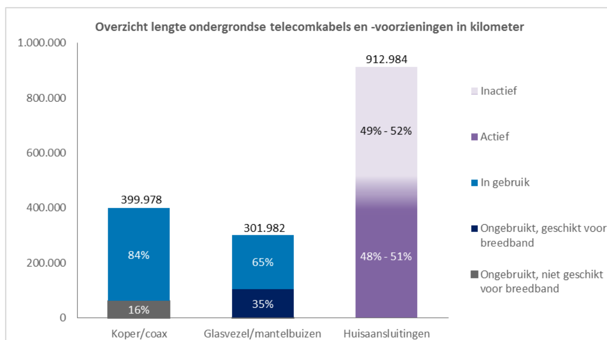
Figuur 14. Totale lengte ondergrondse telecomkabels en -voorzieningen bij de telecomaanhouders die in dit onderzoek data hebben aangeleverd (zie bijlage I).
