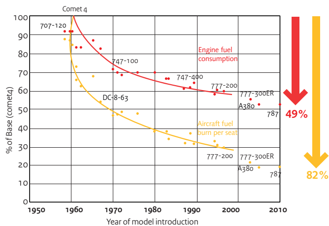
Sinds 1960 is de brandstofefficiëntie van verschillende vliegtuigen sterk verbeterd. Niet alleen het totale brandstofverbruik per vliegtuig is afgenomen, maar ook het brandstofverbruik per stoel.
