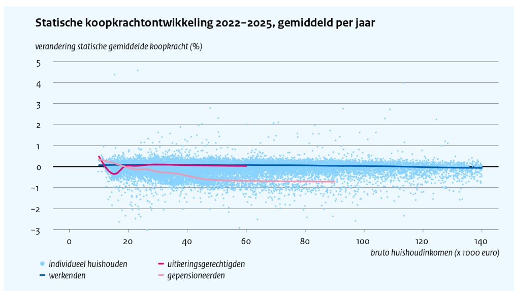
Figuur 3.6 Puntenwolk
